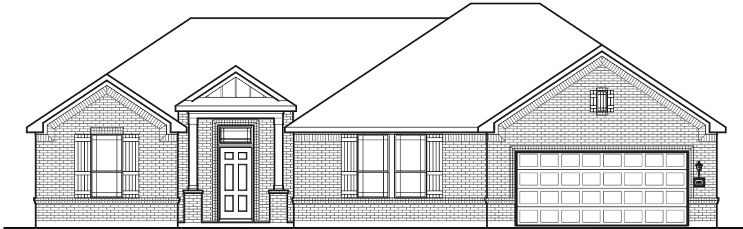
ELEVATION A
