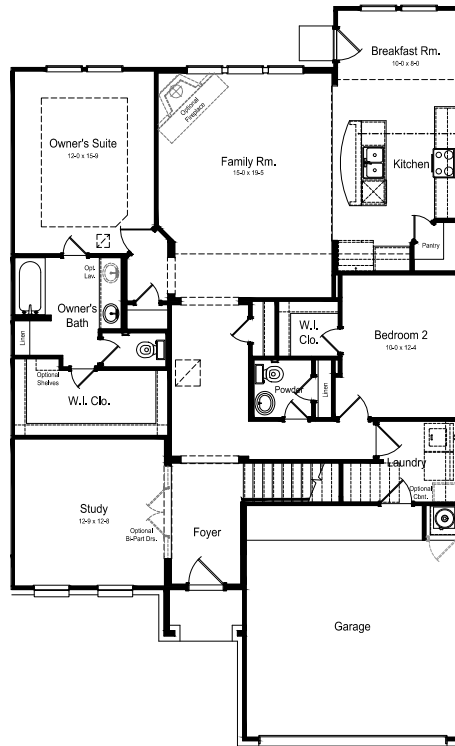
Plan 2648
